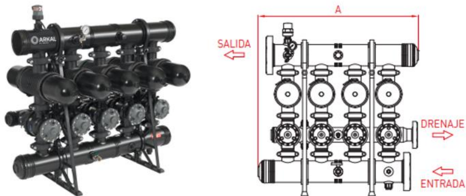
Figura 7. Imagen ilustrativa de los filtros autolimpiantes.
