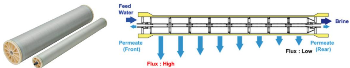
Figura 9. La imagen de la izquierda corresponde al formato de las unidades típicas de una membrana de OI, mientras que la imagen de la derecha representa el sentido de flujo de una membrana.
