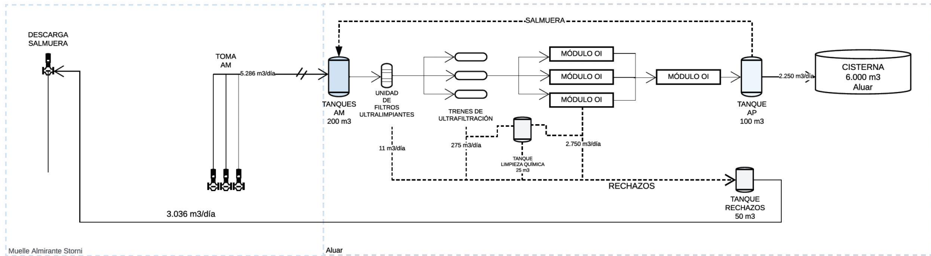
Figura 1. Esquema del proceso del PPOI para una capacidad máxima de producción de AP de 2.250 m³ AP/día.
