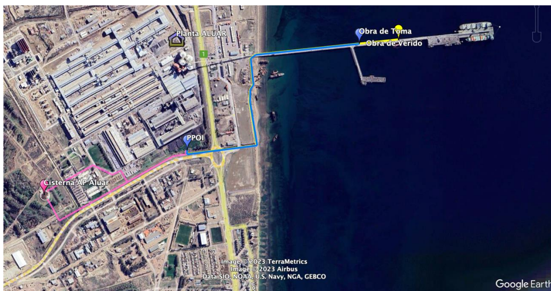
Figura 2. Localización de los principales componentes del PPOI. Obra de Toma y cañería de agua de mar (azul), Obra de vertido y cañería de descarga de salmuera (amarillo), y posibles trazados de cañerías de agua potable hacia cisterna de Aluar (rosa).
