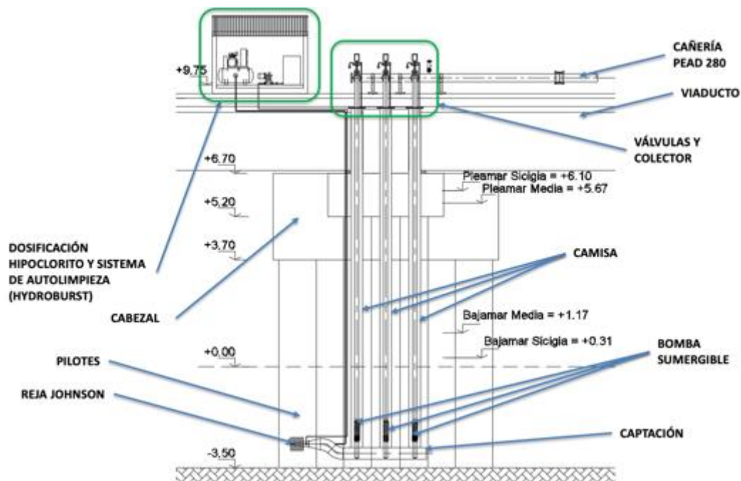
Figura 4. Obra de Toma de AM a instalar sobre el Viaducto del Muelle Almirante Storni, ver Figura 2.
