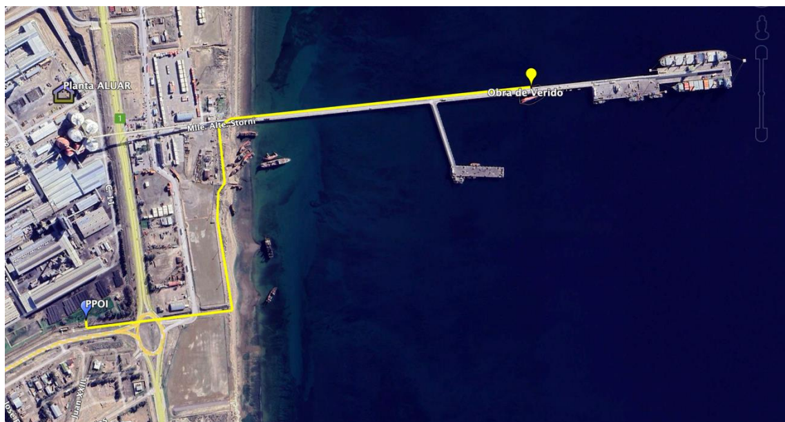
Figura 11. Imagen satelital ubicación de obra de descarga de salmuera al mar y cañería (traza amarilla) de salmuera. Fuente: Google Earth 2023.
