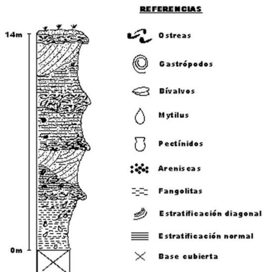
Figura 39. Perfil esquemático de la Formación Puerto Madryn en la estancia La Pastora.
