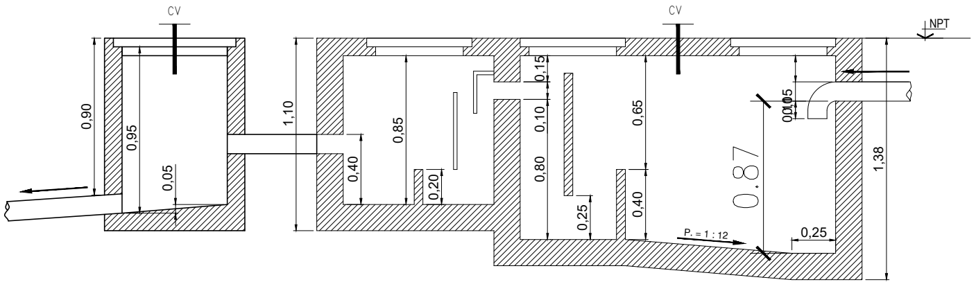
CORTE: 1-1
