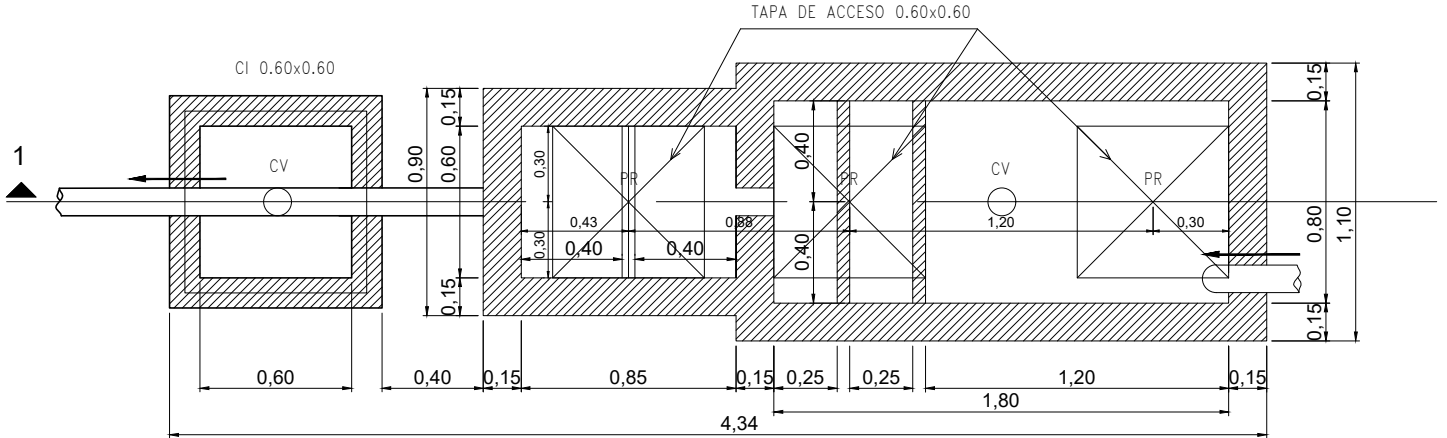
PLANTA
